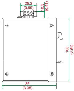
左侧视图
