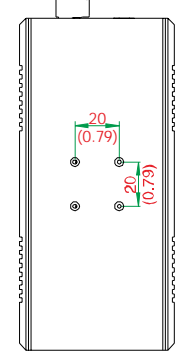
后视图
