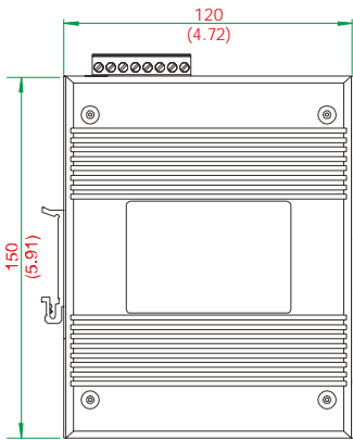
左侧视图
