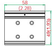
导轨片
