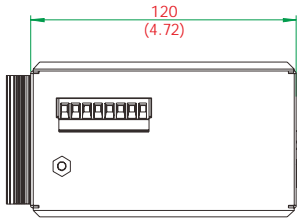
顶视图
