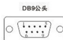
RS-232公头引脚定义:
